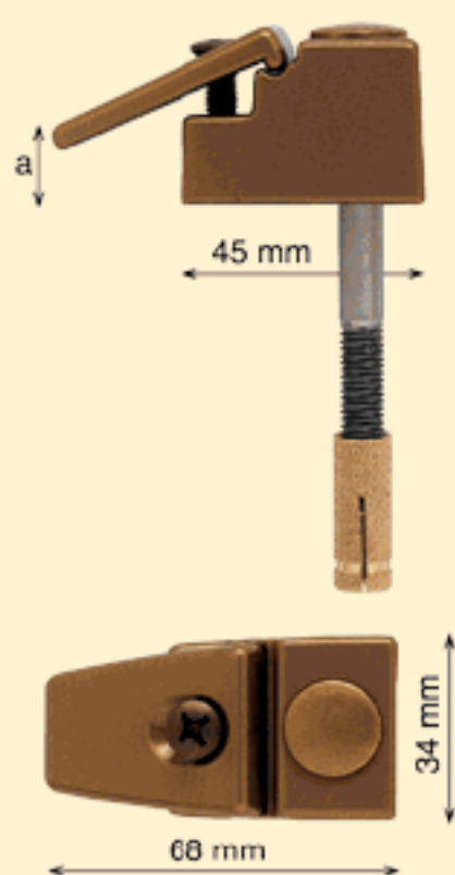
Art. 30783A a =cm. 1-2 Tornillo inox con hexágono insertado + taco de latón M8 incluido en el precio
