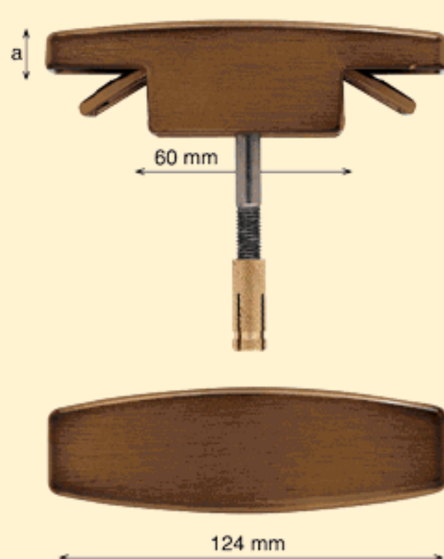
Art. 30781A a =cm. 1-2 Tornillo inox con hexágono insertado + taco de latón M8 incluido en el precio
