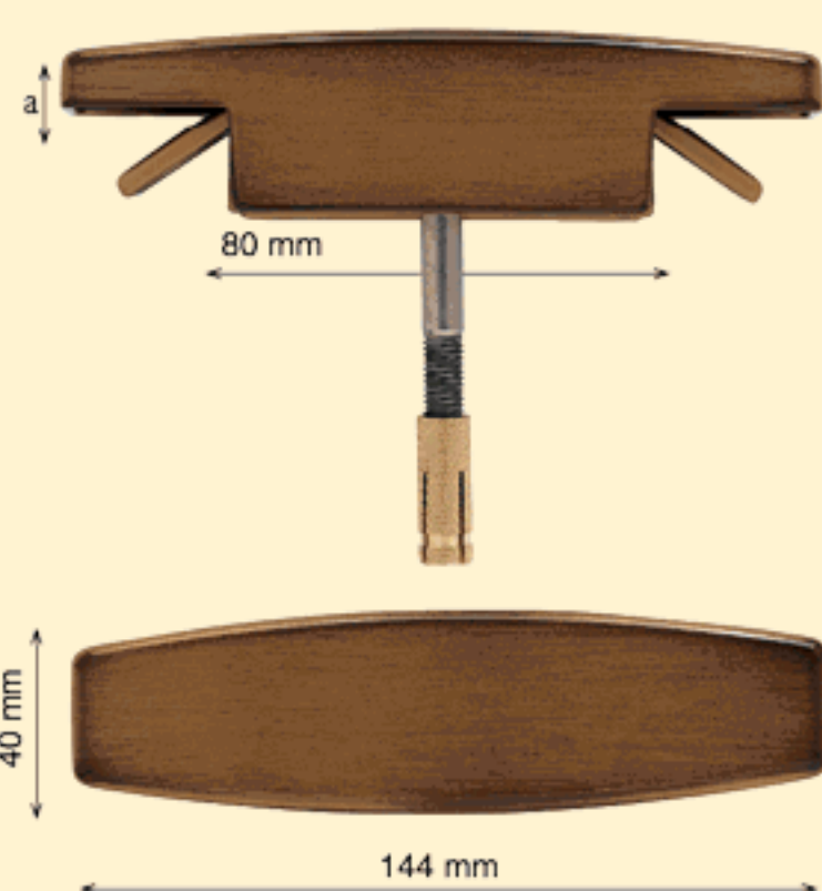
Art. 30782A a =cm. 1-2 Tornillo inox con hexágono insertado + taco de latón M8 incluido en el precio
