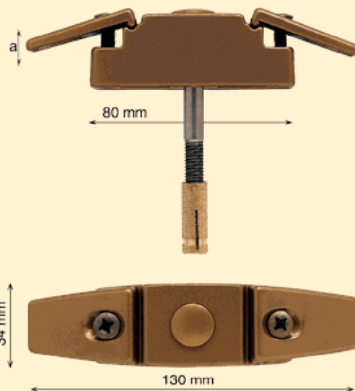
Art. 30785A a =cm. 1-2 Tornillo inox con hexágono insertado + taco de latón M8 incluido en el precio
