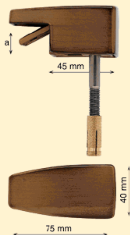
Art. 30780A a =cm. 1-2 Tornillo inox con hexágono insertado + taco de latón M8 incluido en el precio
