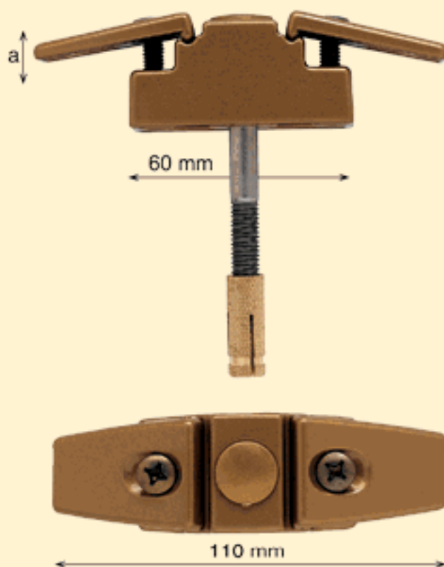
Art. 30784A a =cm. 1-2 Tornillo inox con hexágono insertado + taco de latón M8 incluido en el precio
